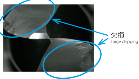
従来ボールエンドミル2刃 0.7m加工後 Conventional 2-flute ball end mill After milling 0.7m
