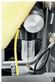
ウォーターセパレーター
