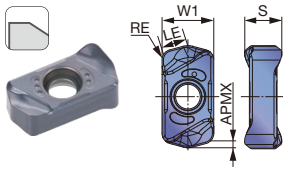
LNMU03ZER-MS (ステンレス用ブレード)
