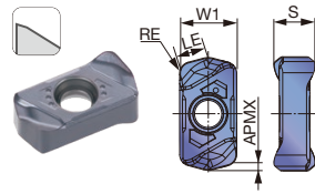
LNGU03ZER-MH (対先強化型ブレード)
