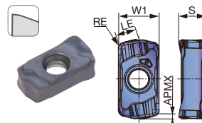
LNMU03UER-ML (低切込み角、低抵抗ブレード)
