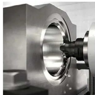
CoroMill® MS60
