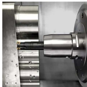
CoroMill® MS40
